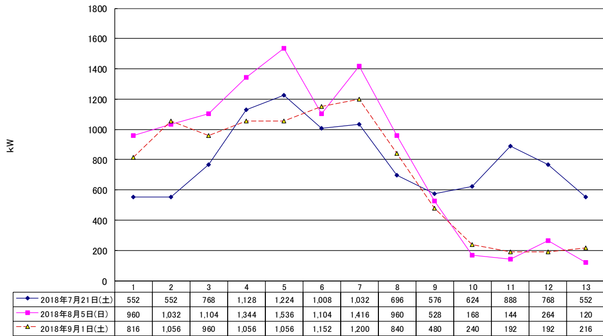
平成30年 夏季最大使用指定日の需給カーブ
