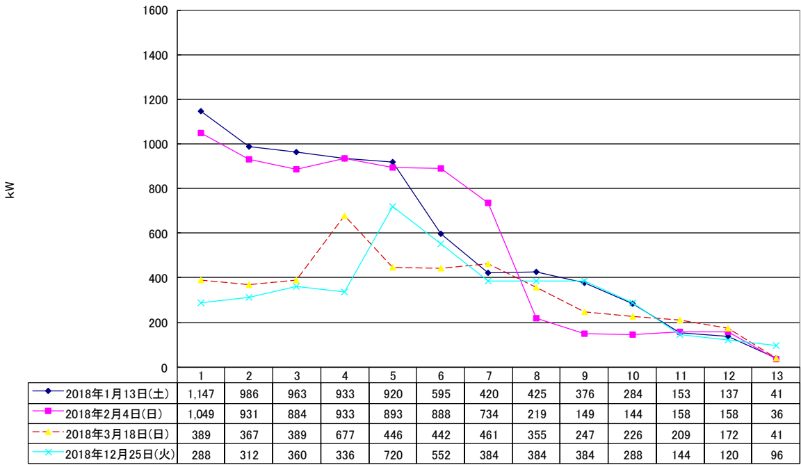
平成30年 冬季最大使用指定日の需給カーブ
